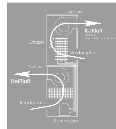
Klimagerät für 25 oder 50 m 3 Ableitungsseite für Kaltluft
